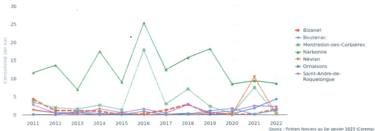
Comparaison de la consommation annuelle d'espace entre Bizanet et les territoires similaires entre 2011 et 2022 (en ha)
